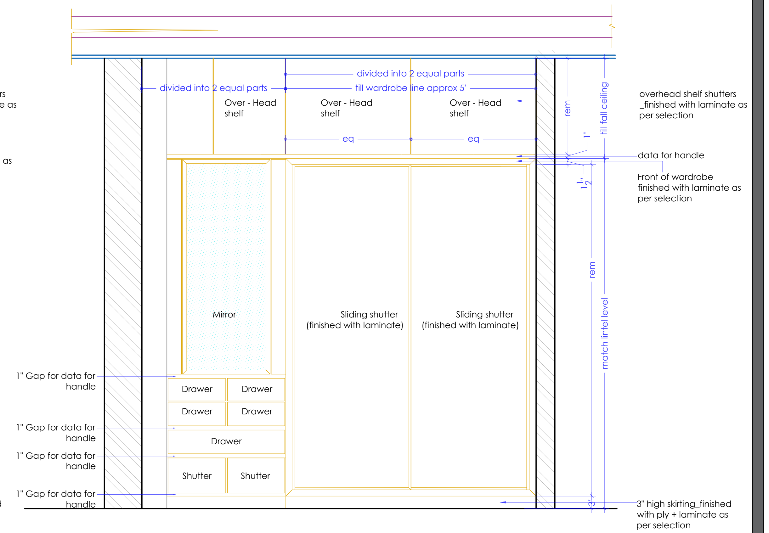
ELEVATION
